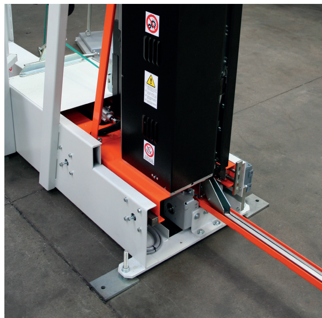
Palettenlanze um durch Palettendeck zu umreifen
